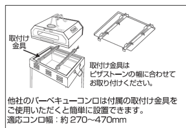
設置方法
